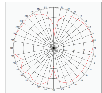
1.9 GHz
