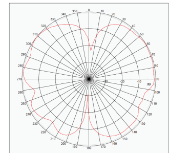
1.575 GHz
