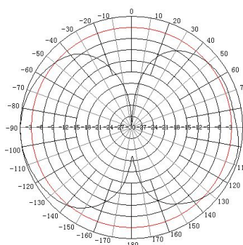
E-Plane: 700-960MHz
