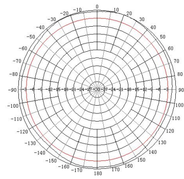
H-Plane: 1710-2700MHz
