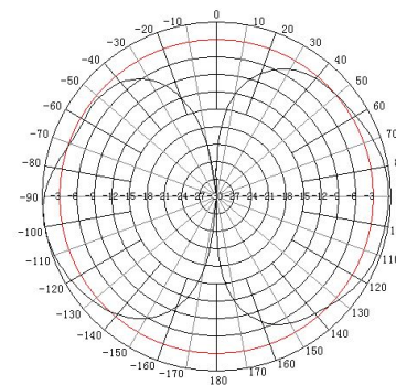
E-Plane: 1710-2700MHz
