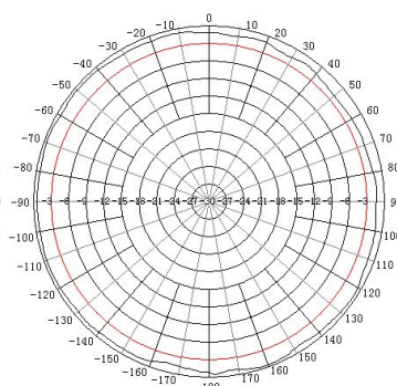
H-Plane: 700-960MHz
